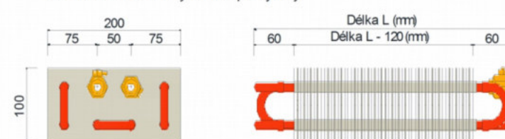
FCVT8-200-100-01 Výměník tepla čtyřřadý
