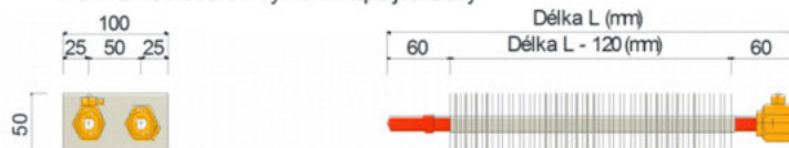
FCVT3-100-100-01 Výměník tepla dvouřadý
