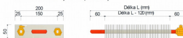
FCVT4-200-050-01 Výměník tepla dvouřadý
