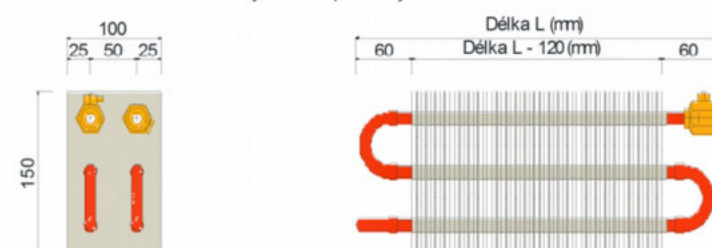
FCVT6-150-100-01 Výměník tepla třířadý
