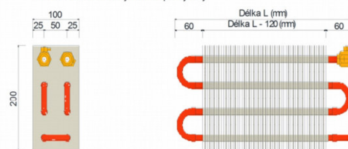
FCVT8-200-100-01 Výměník tepla čtyřřadý
