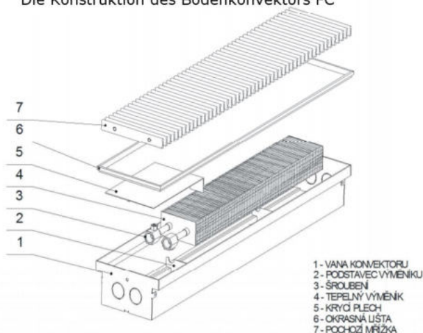
Die Konstruktion des Bodenkonvektors FC
