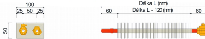
FCVT3-100-100-01 Výměník tepla dvouřadý
