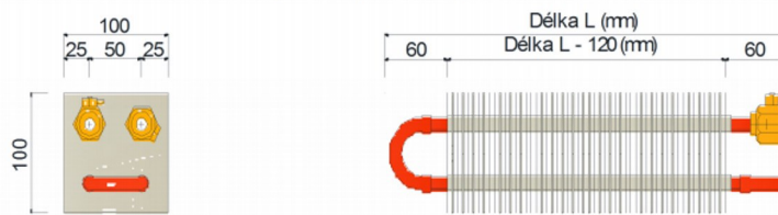
FCVT4-200-050-01 Výměník tepla dvouřadý
