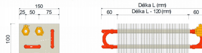
FCVT6-150-100-01 Výměník tepla třířadý
